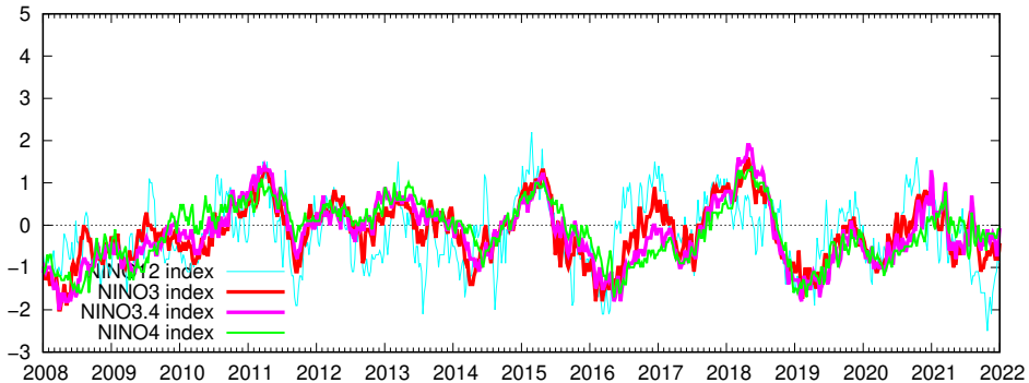
CPC/NCEP ENSO indices
